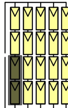
2 árnyékolt napelem = 1 sor
