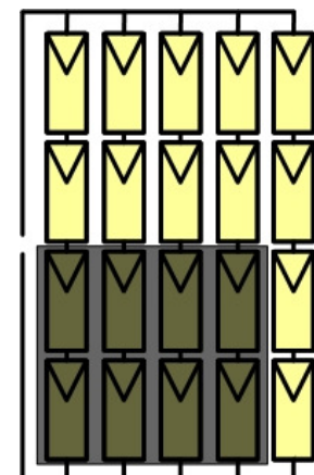
8 árnyékolt napelem = 4 sor
