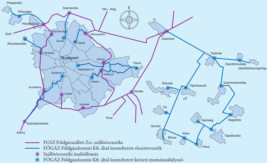
A FŐGÁZ Földgázelosztási Kft. által üzemeltetett 5 848 km hosszú gázelosztó hálózat összetétele 2010. december 31-én
